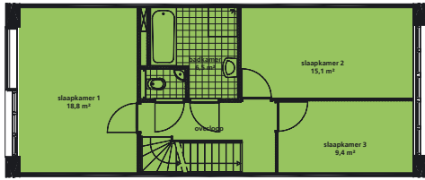
eerste verdieping
